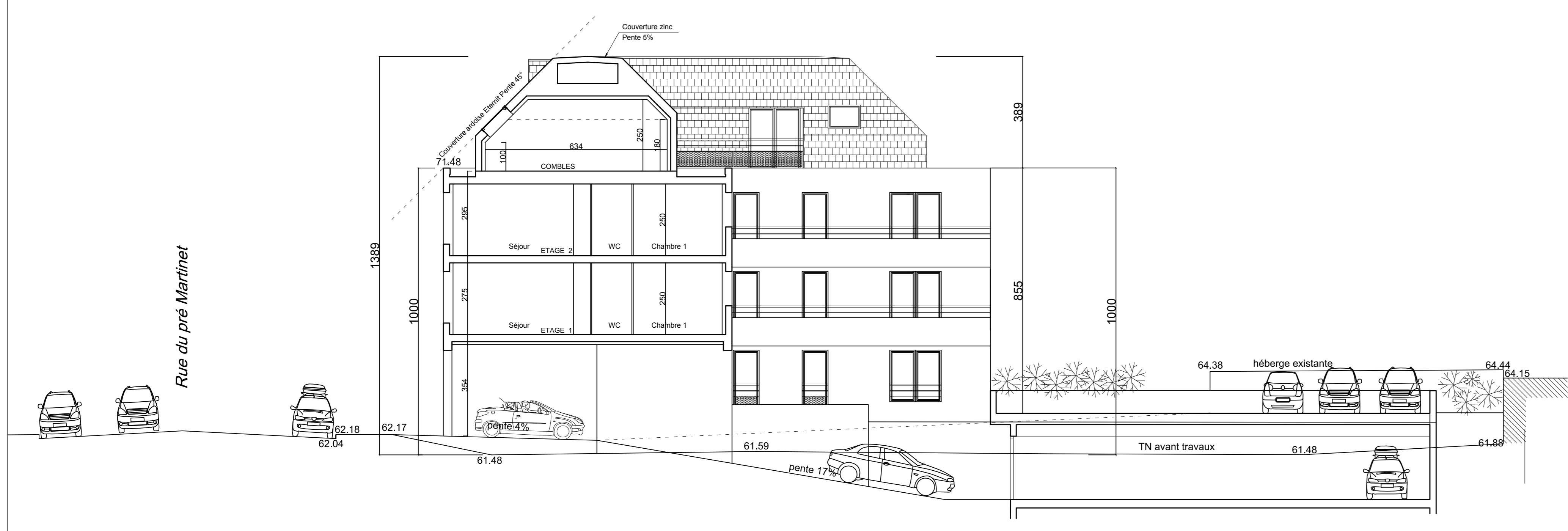
PC3 - Coupe sur porche
