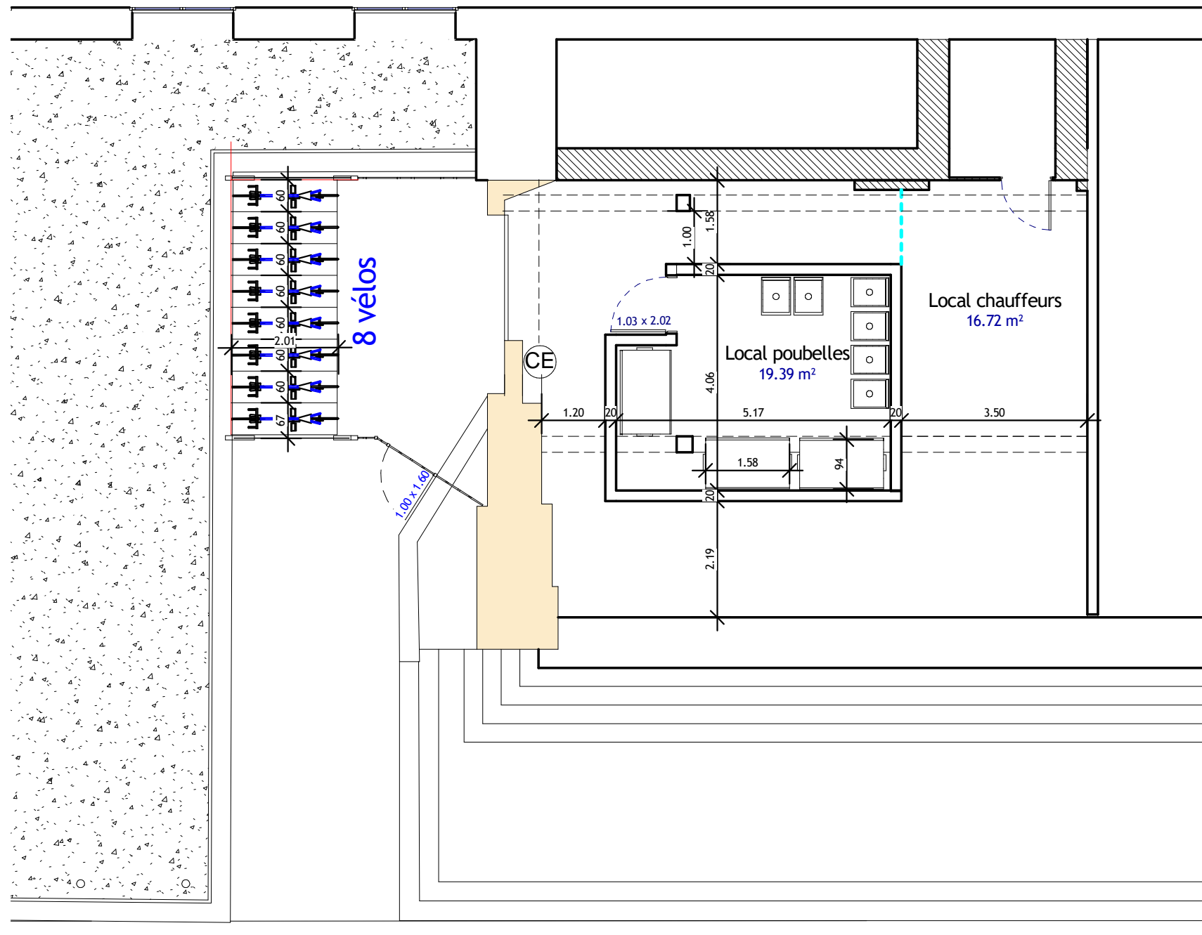
1 LOCAL POUBELLES + VELOS Ech : 1 : 100
