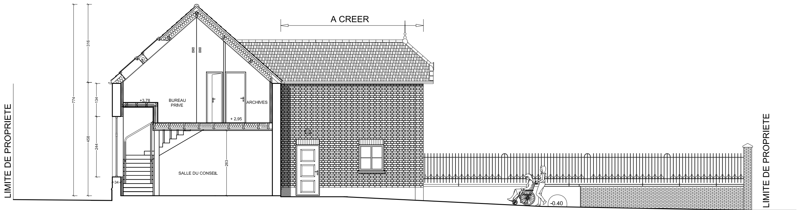
COUPE LONGITUDINALE SUR LE TERRAIN
